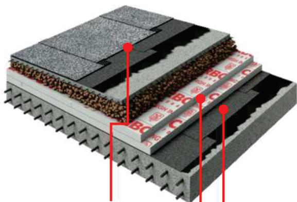
PRIMA PLAST PV - 2 lớp Xốp cách nhiệt Màng tự dính BITUMAX 1.5mm
